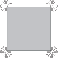
Format 60 x 60 cm 4 Auflagepunkte je Platte 3,4 Stück/m 2
