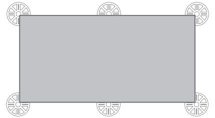
Format 60 x 120 cm 6 Auflagepunkte je Platte 3,4 Stück/m 2
