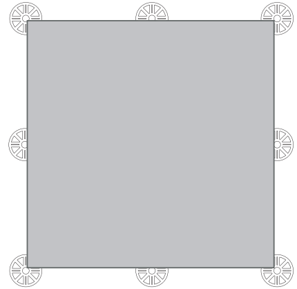
Format 120 x 120 cm 8 Auflagepunkte je Platte 2,7 Stück/m 2
