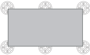
Format 45 x 90 cm 6 Auflagepunkte je Platte 6 Stück/m 2
