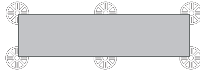
Format 30 x 120 cm 6 Auflagepunkte je Platte 7 Stück/m 2
